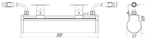
Рисунок 1 Светильник «L-contour 300».
